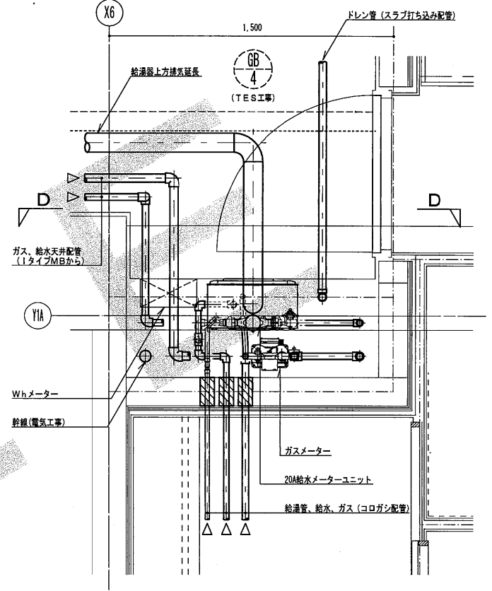
給排水衛生設備JタイプMB詳細図
