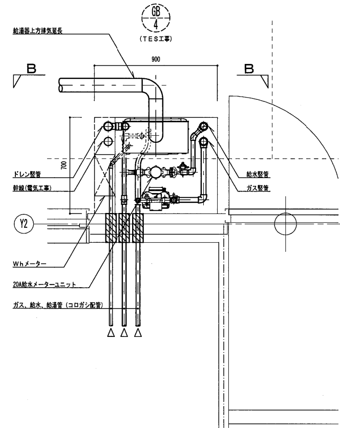
給排水衛生設備Fタイプ1~2階MB詳細図
