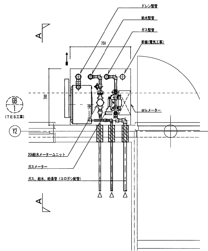
給排水衛生設備EタイプMB詳細図
