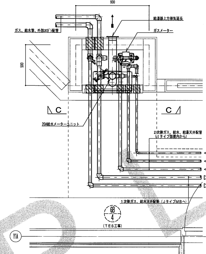
給排水衛生設備IタイプMB詳細図
